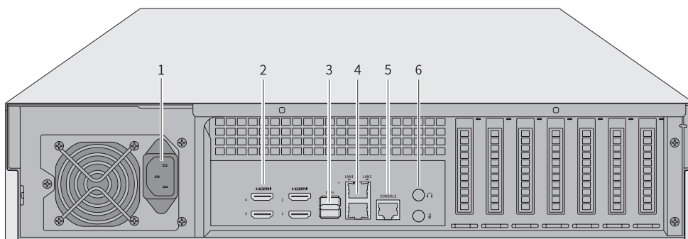
图1-3 TL-TUMS2500-N-A后面板示意图
