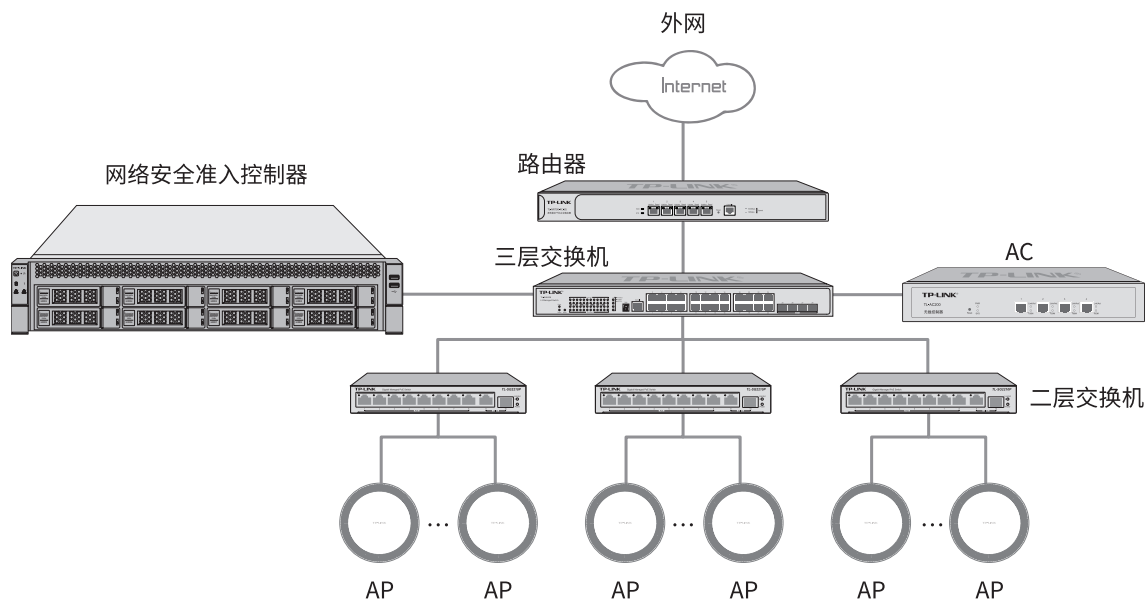
图3-1 设备连接示意图
